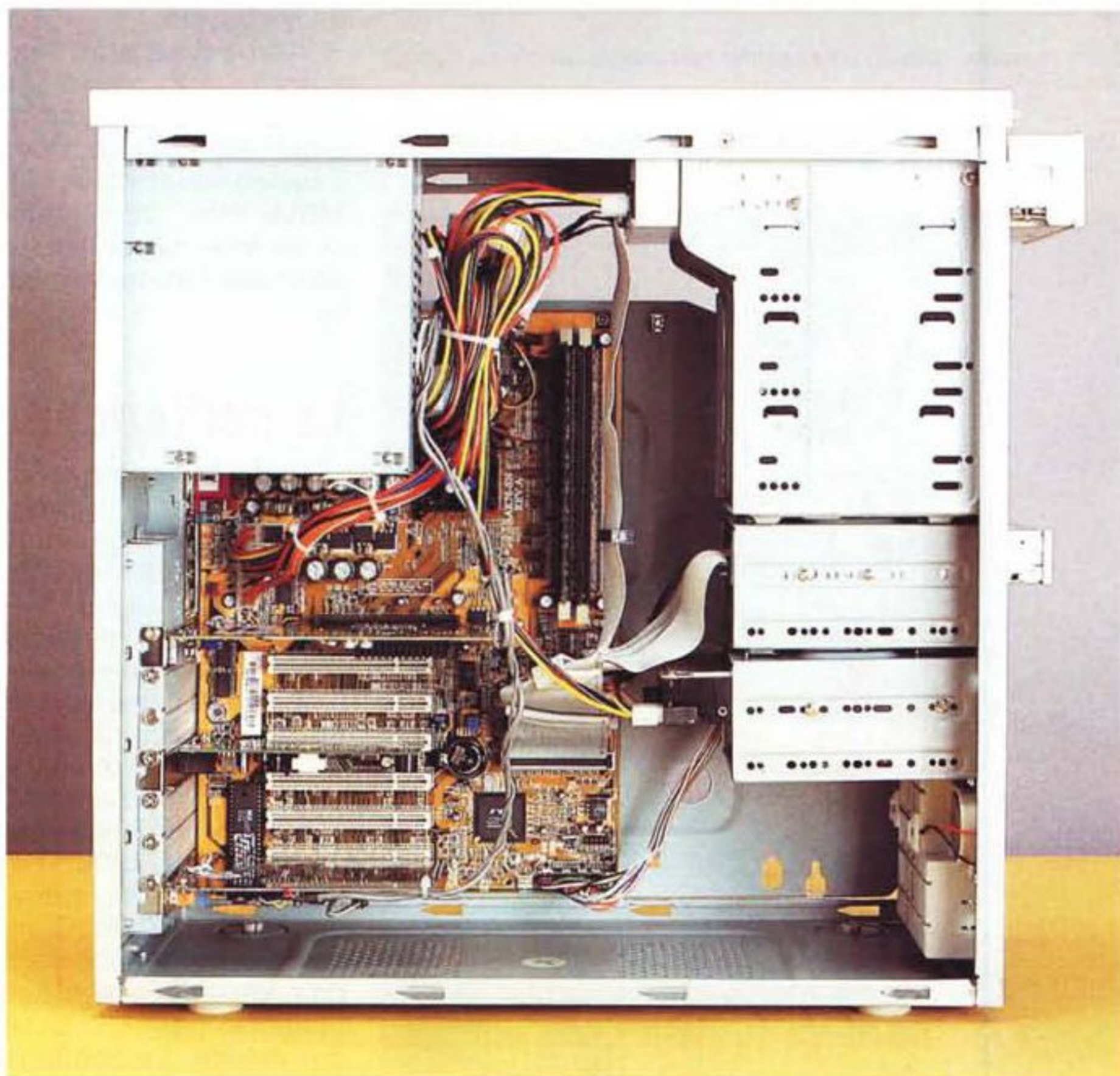
Vista d'insieme all'interno del cabinet.
