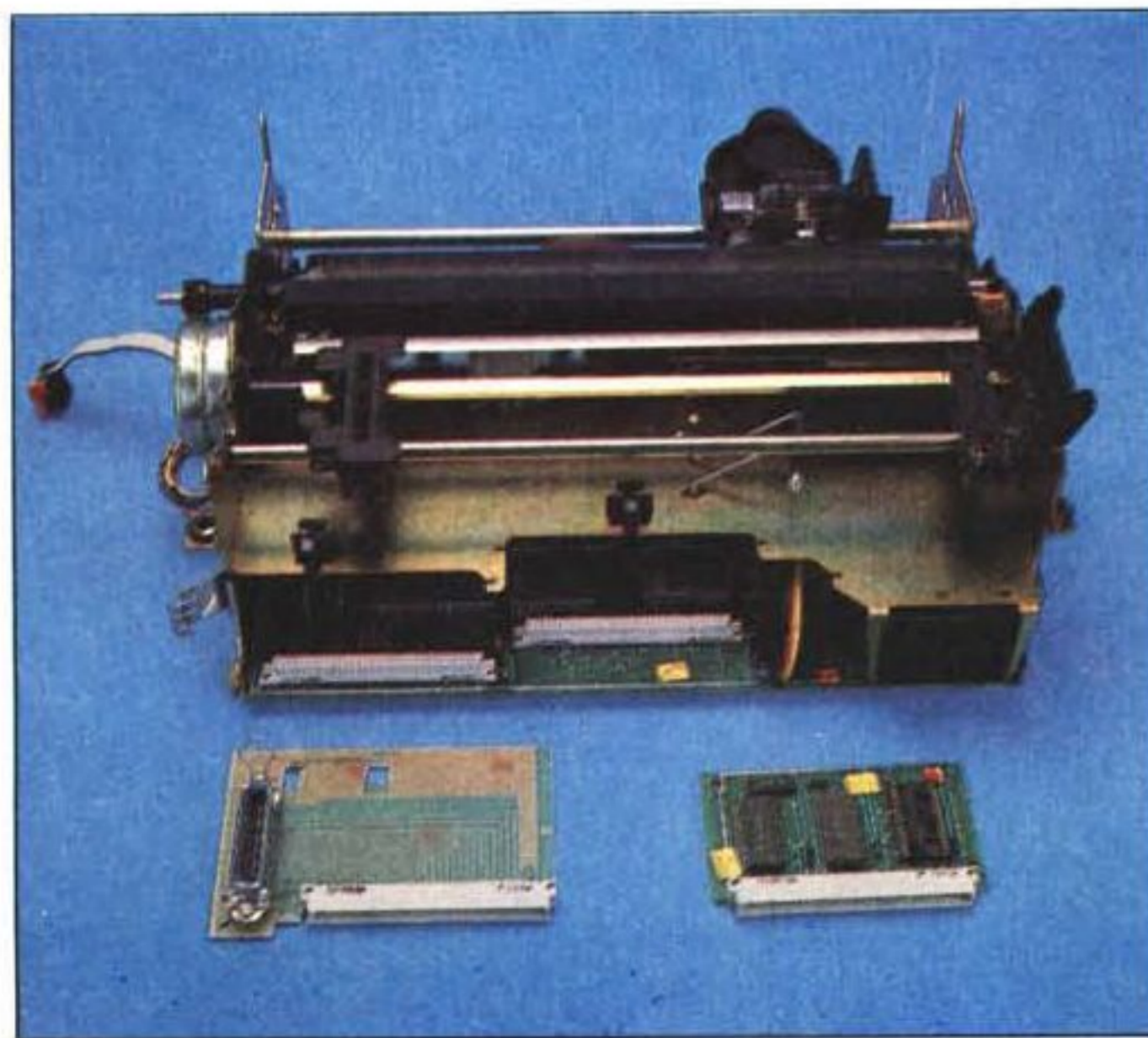
Due viste posteriori dello chassis, dedicate all'elettronica. A sinistra vediamo le due schede del connettore e del generatore di caratteri estratte dai propri connettori. A destra un particolare della piastra madre.
