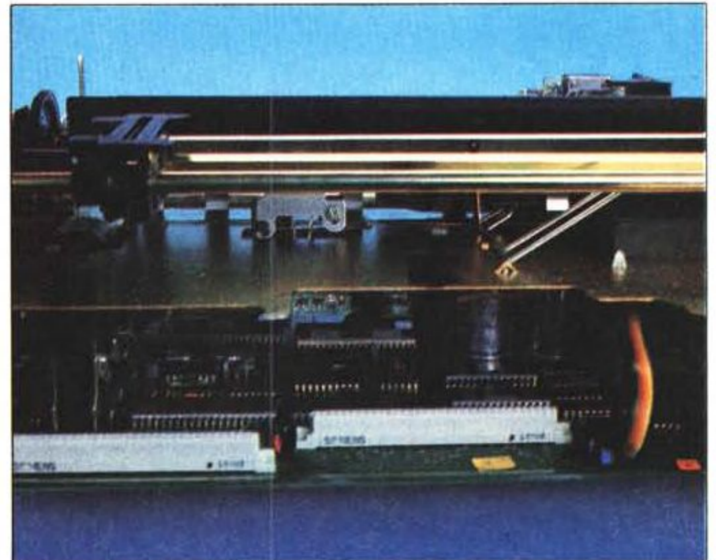
Due viste posteriori dello chassis, dedicate all'elettronica. A sinistra vediamo le due schede del connettore e del generatore di caratteri estratte dai propri connettori. A destra un particolare della piastra madre.
