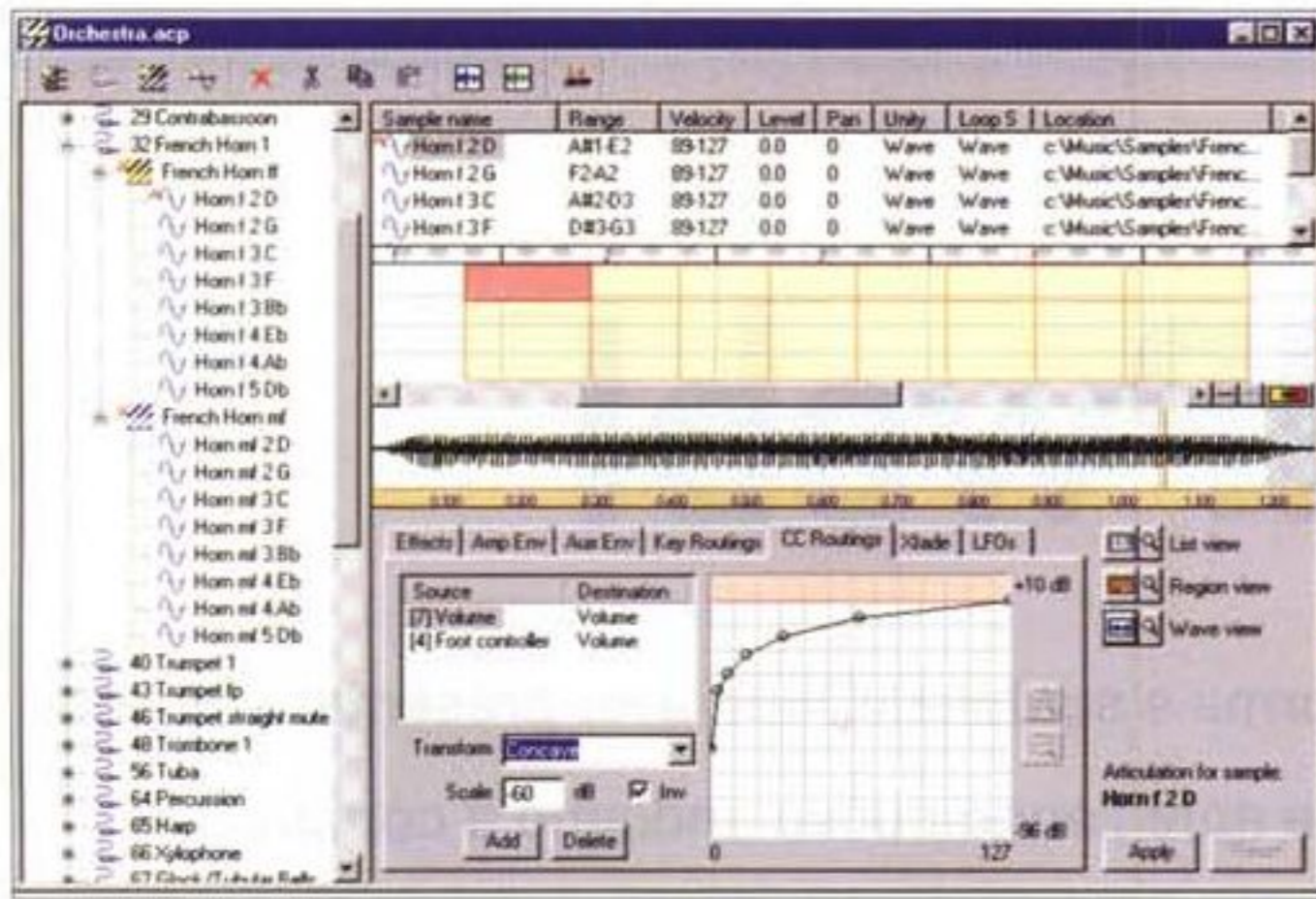
Audio Composer: modalità Patch Editor nella quale è possibile operare alla visualizzazione e alle modifiche dei parametri qualitativi dei campioni sonori.
