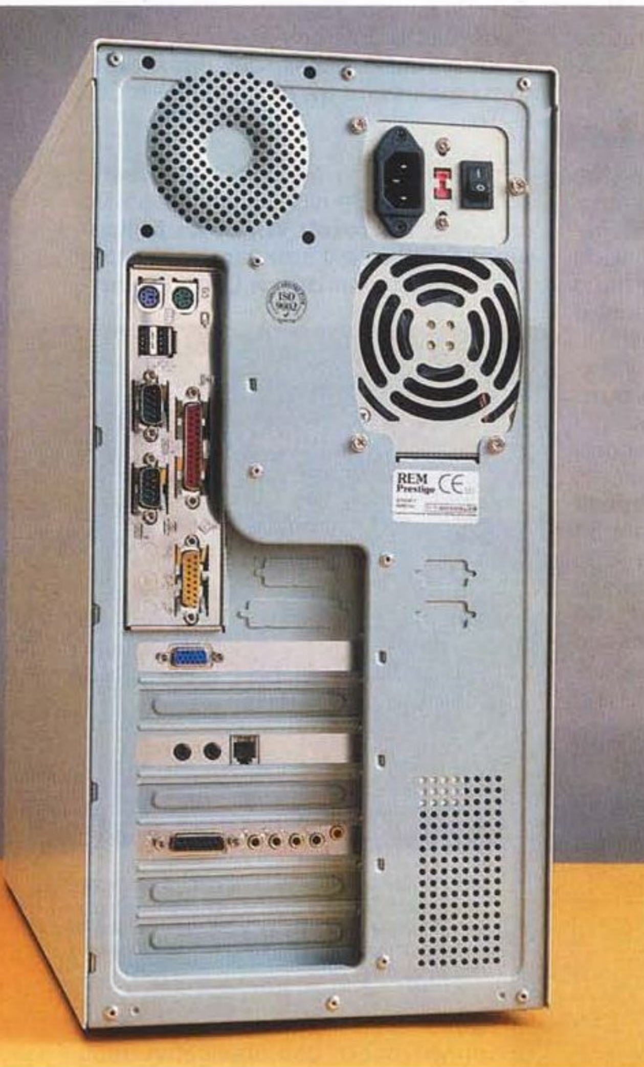
Vista del retro del REM Prestige. Da notare che oltre alle usuali connessioni offerte della SoundBlaster Live!, sulla scheda madre FastFrame è presente un chip on-board per la codifica AC97 che controlla altre linee I/O. Queste vengono comunque, disabilitate al momento dell'inserzione della scheda audio.
