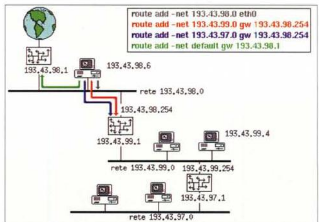
Figura 1: Schema relativo all'esempio di rete proposto.
