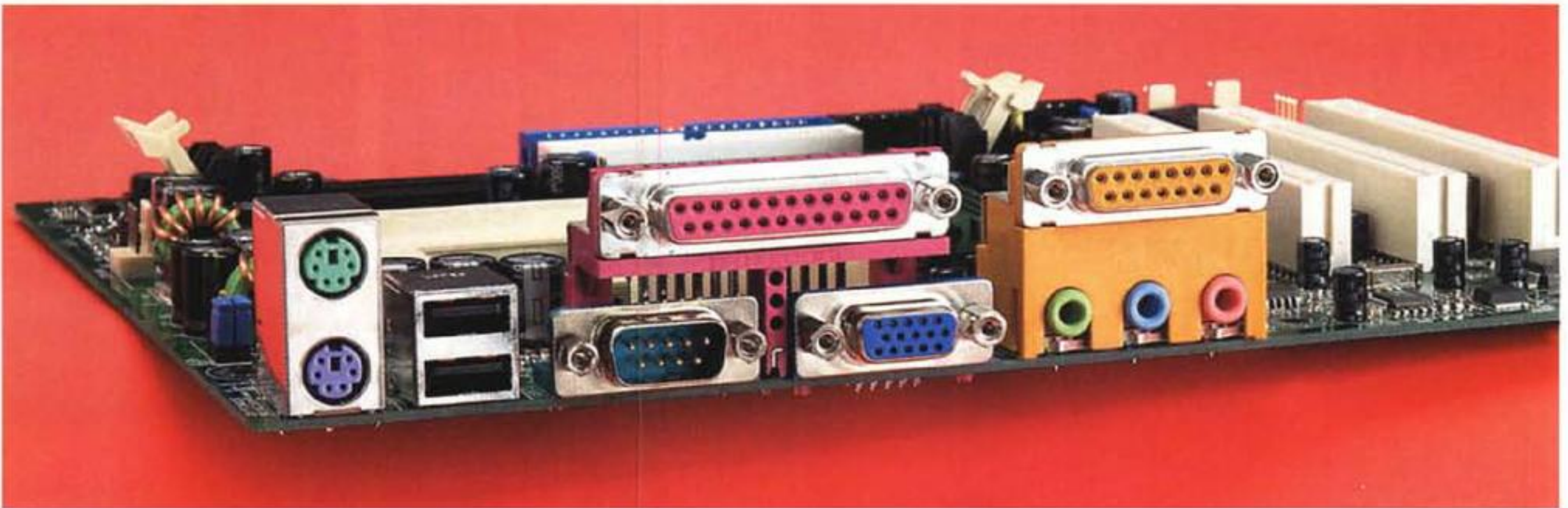
Le porte di I/O della scheda madre: la disposizione e la colorazione seguono le specifiche PC99; si noti, al posto della seconda porta seriale, la presenza del connettore VGA.
