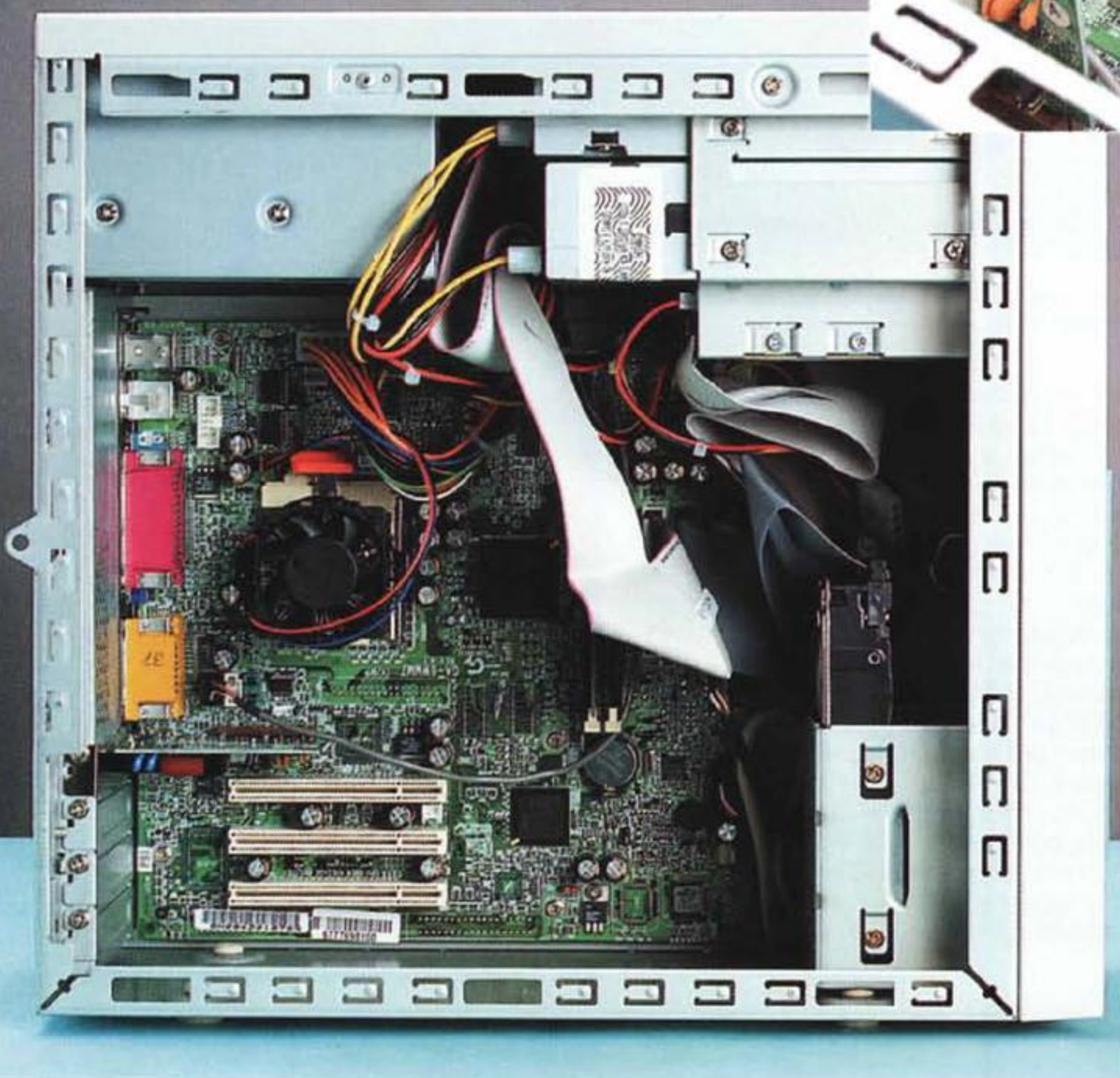
Vista d'insieme dell'interno: malgrado la sensazione sia quella di una scheda madre assolutamente deserta, in realtà, proprio on-board l'iconnect 1700 RW possiede già presenti chip audio e acceleratore grafico, gestiti attraverso il chipset i810-L (100Mhz), il quale compie al meglio il suo dovere.
