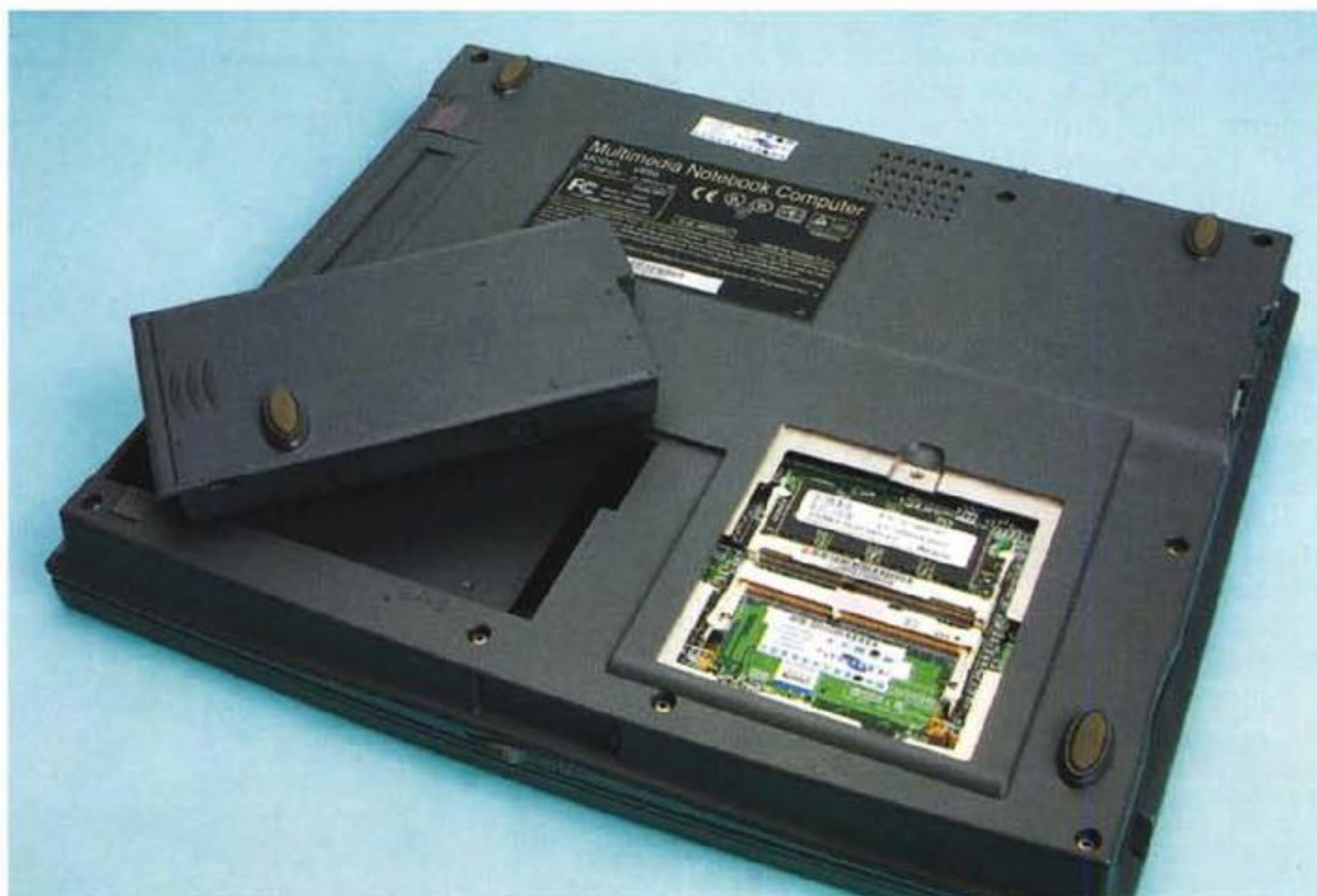
Sul lato inferiore troviamo l'ampio e comodo vano memoria, dotato di una vite di protezione, facilmente accessibile per le eventuali operazioni di ampliamento della SDRAM. Possiamo da qui inoltre accedere ai nottolini di sblocco della batteria agli ioni di litio e dell'unità DVD-ROM.
